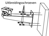
Afbeeldingen 1-6 De muurmontagebeugel monteren
