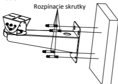
Obrázok 1-6 Namontujte stenovú montážnu konzolu
