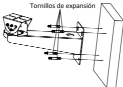
Figura 1-6 Instalación del soporte de montaje en pared
