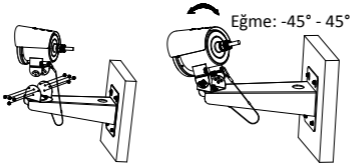
Şekil 1-10 Kameranın Duvara Montaj Braketine Sabitlemesi
