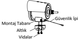
Şekil 1-8 Kameranın Altlığı Sabitlemesi
