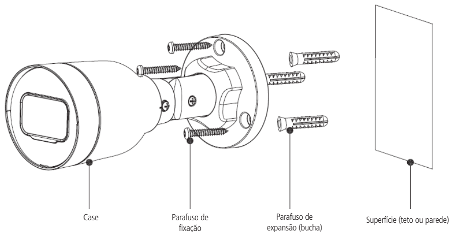
Vista detalhada VIP 1130 B e VIP 1230 B
