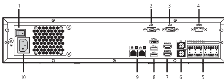
Panel posterior
