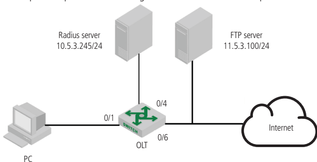
Diagrama de rede para exemplo de configuração de raio
