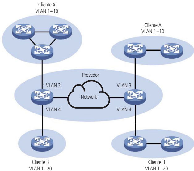
Aplicação QinQ
