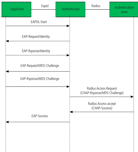
Processo de autenticação EAP-Transfer
